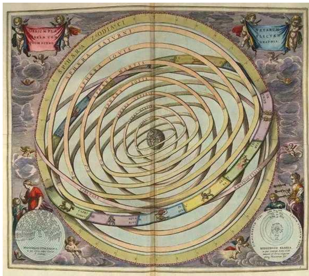
Геоцентрическая модель Птолемея
