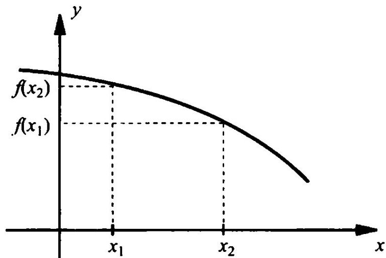
Убывающая функция f(x_2) < f(x_1)
