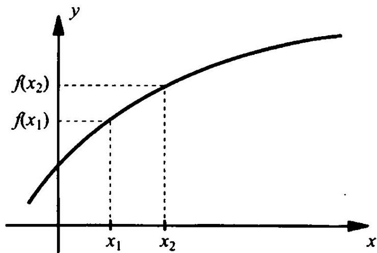
Возрастающая функция f(x_2) > f(x_1)
