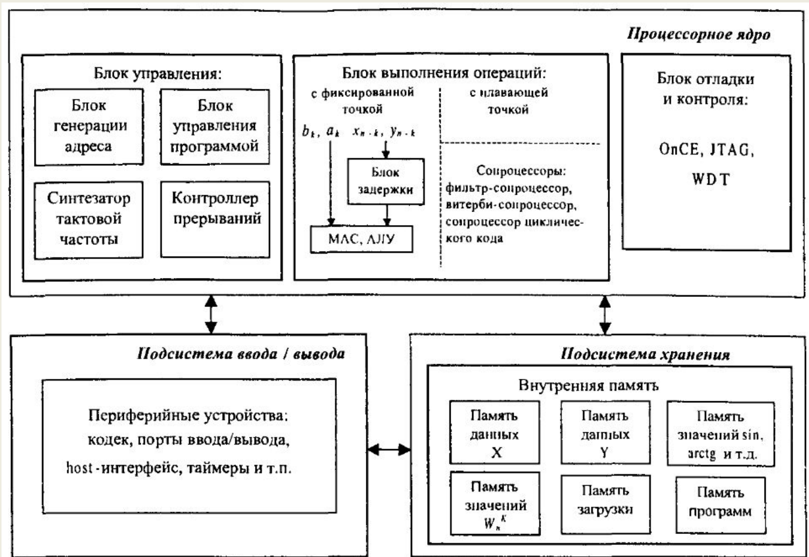
Рис. 2 – Обобщенная архитектура ЦСП
