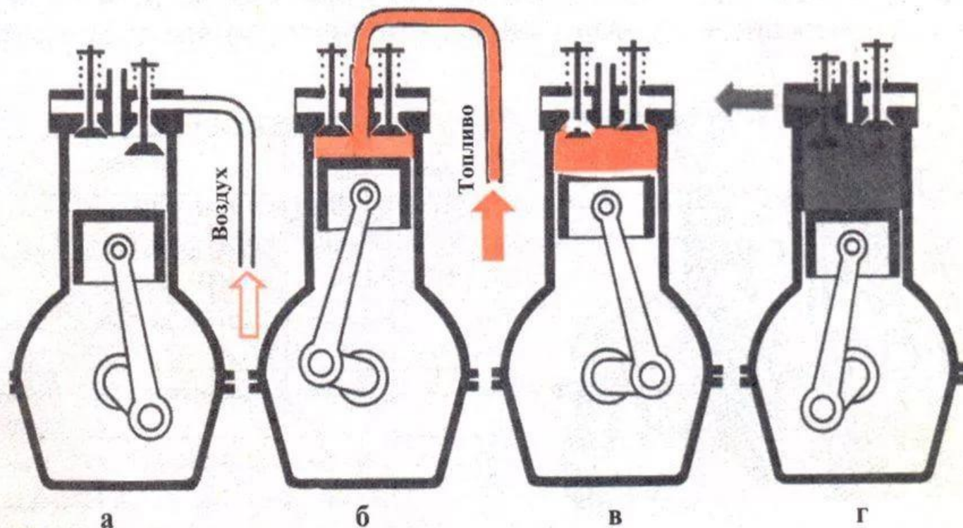
Рис. 7. Схема работы четырехтактного одноцилиндрового дизеля:
