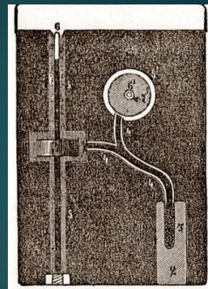
Схема метательного снаряда конструкции Кибальчича (из материалов следствия)
