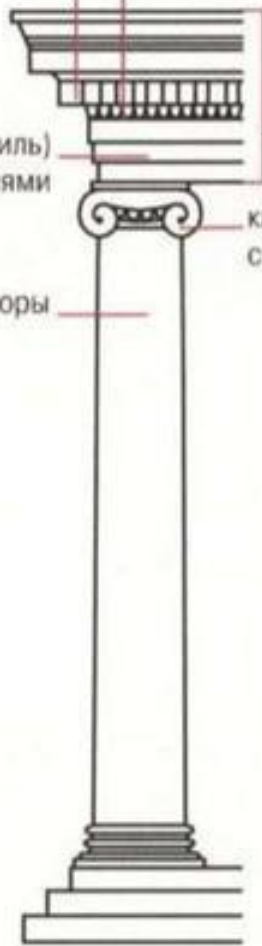
Ионический ордер
