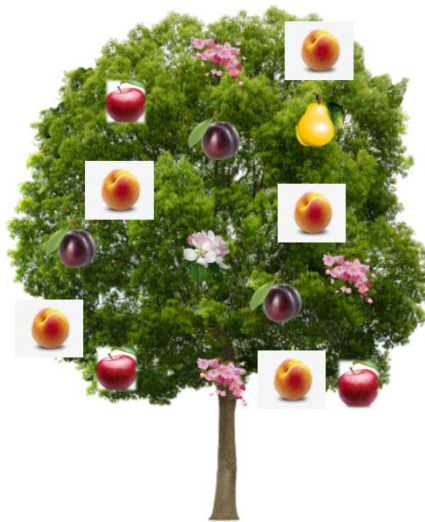
Дерево отряда
