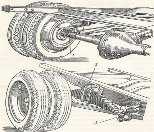
Фиг. 397. Установка задних рессор автомобилей ГАЗ-АА и ГАЗ-ММ.
