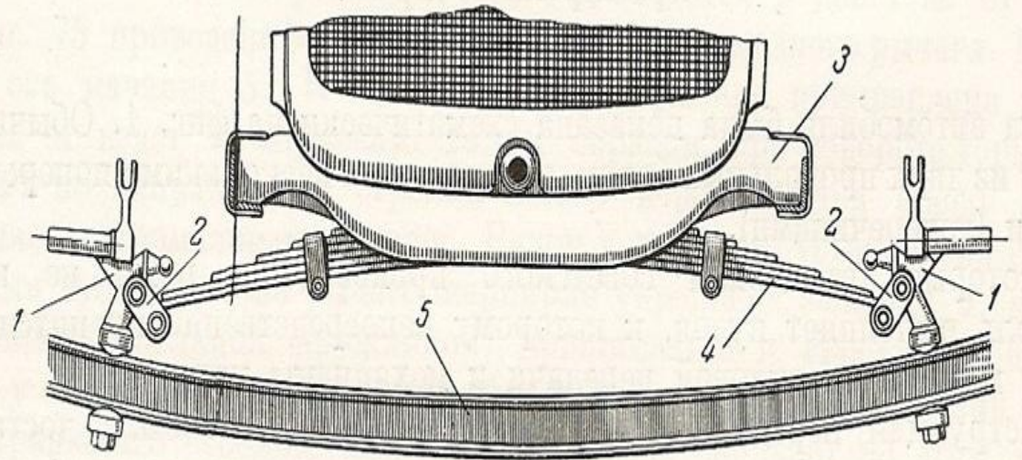
Фиг. 78. Установка передней поперечной рессоры на автомобилях ГАЗ-А и ГАЗ-АА.
