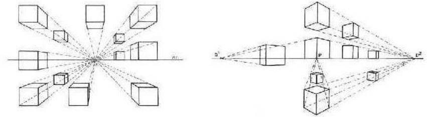
Перспективы куба во фронтальном и угловом положениях
