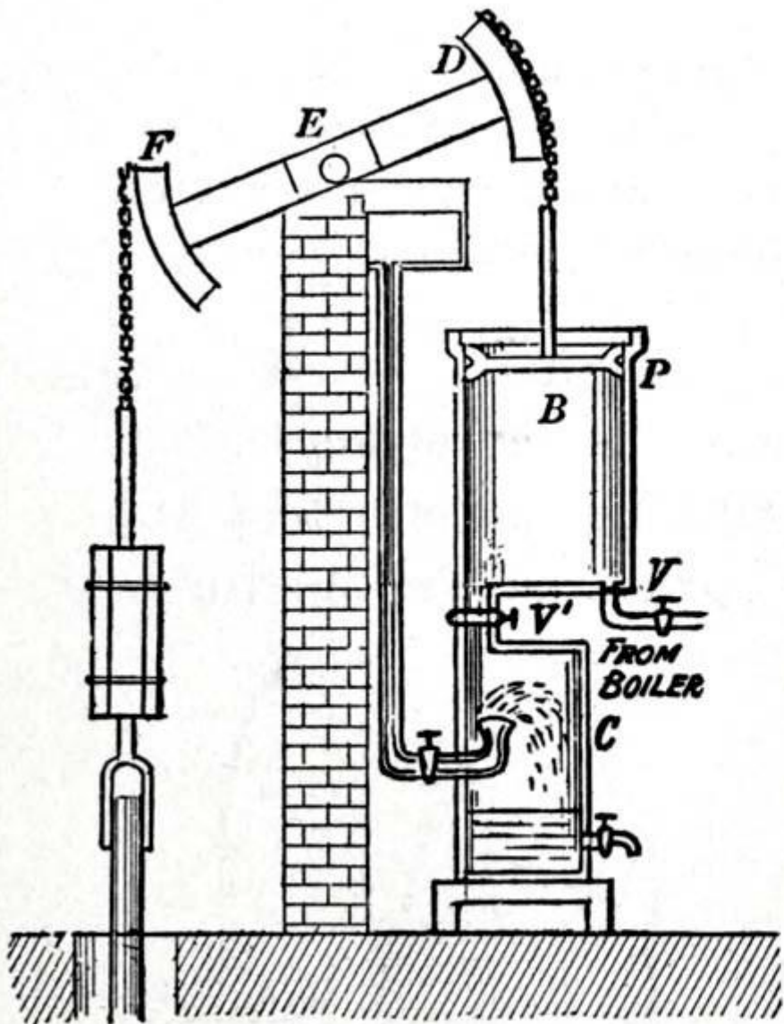
Паровая машина Джеймса Уатта
