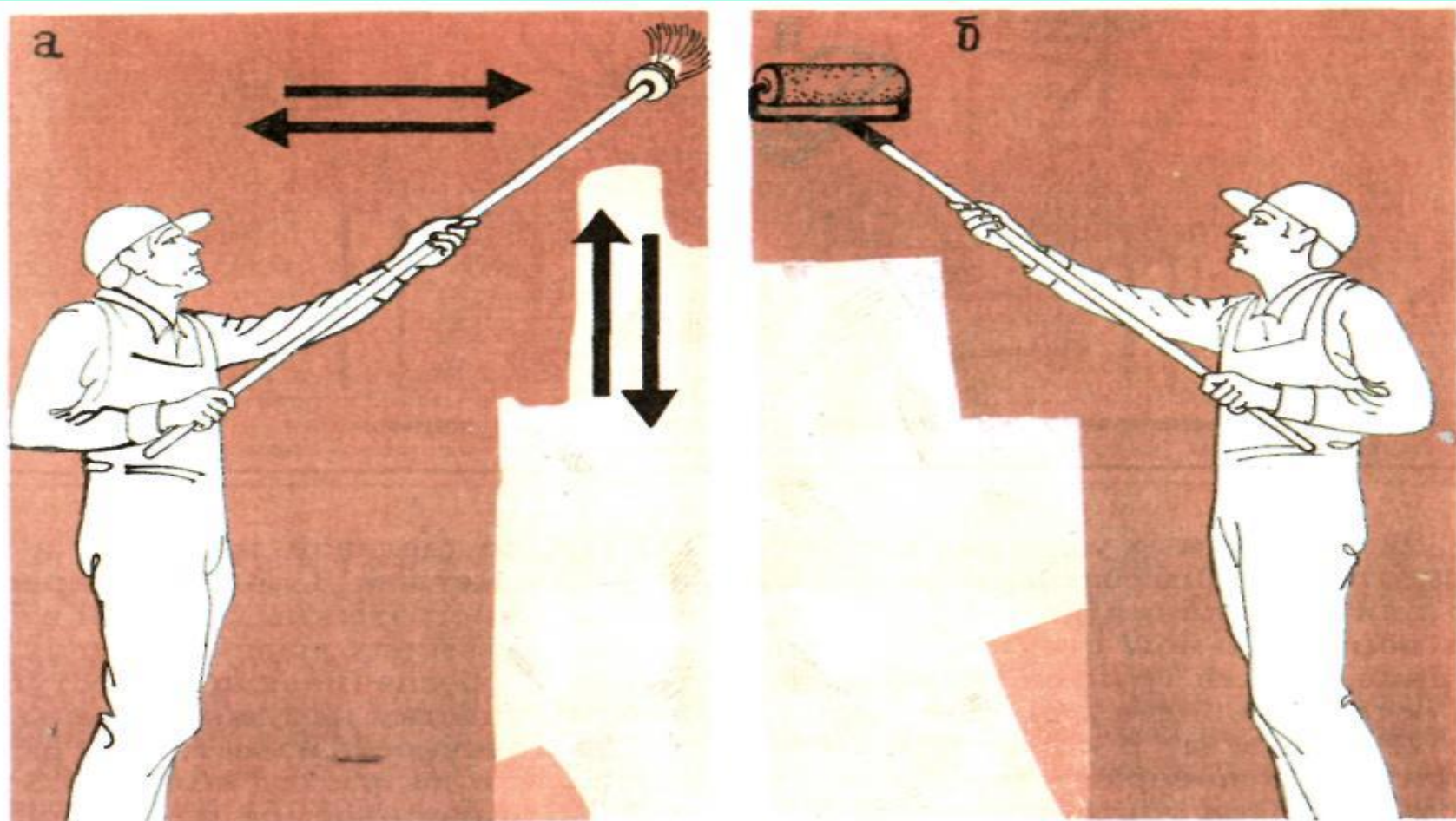
Рис. 249. Окраска фасадов а — маховой кистью; б — валиком
