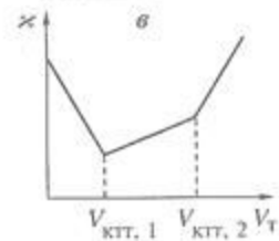
Титрование смеси двух кислот сильным основанием
