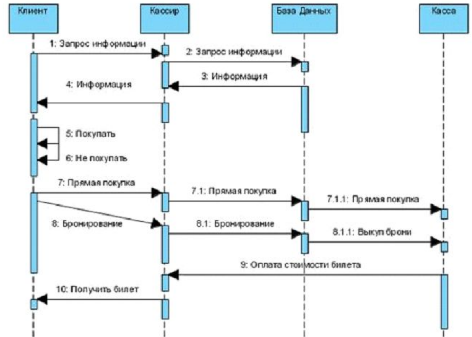
Диаграмма последовательностей
