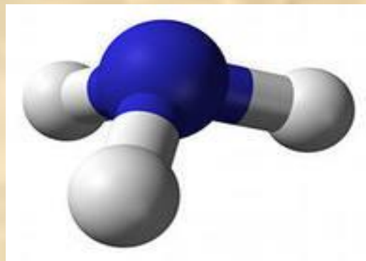
Аммиак \text{NH}_3
