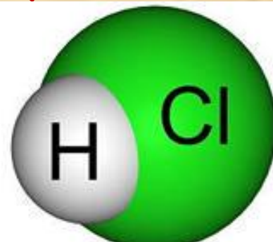
Хлороводород HCl
