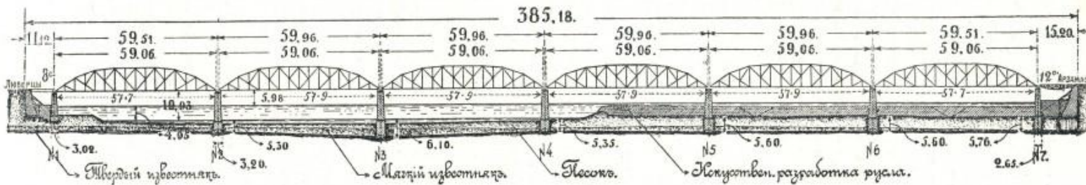
Черт. № 8 Схема моста съ геологическимъ разрѣзомъ.
