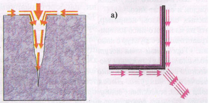
Рис. 69. Вспучивание пространства
