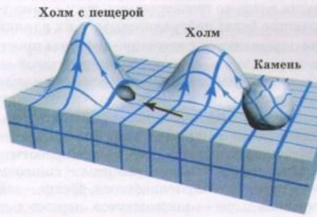
Рис. 69. Вспучивание пространства
