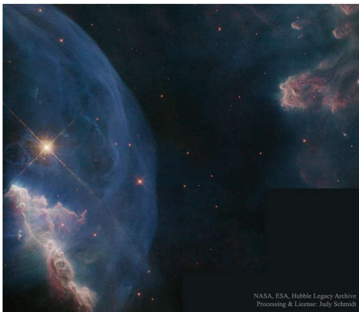
Туманність Бульбашка
