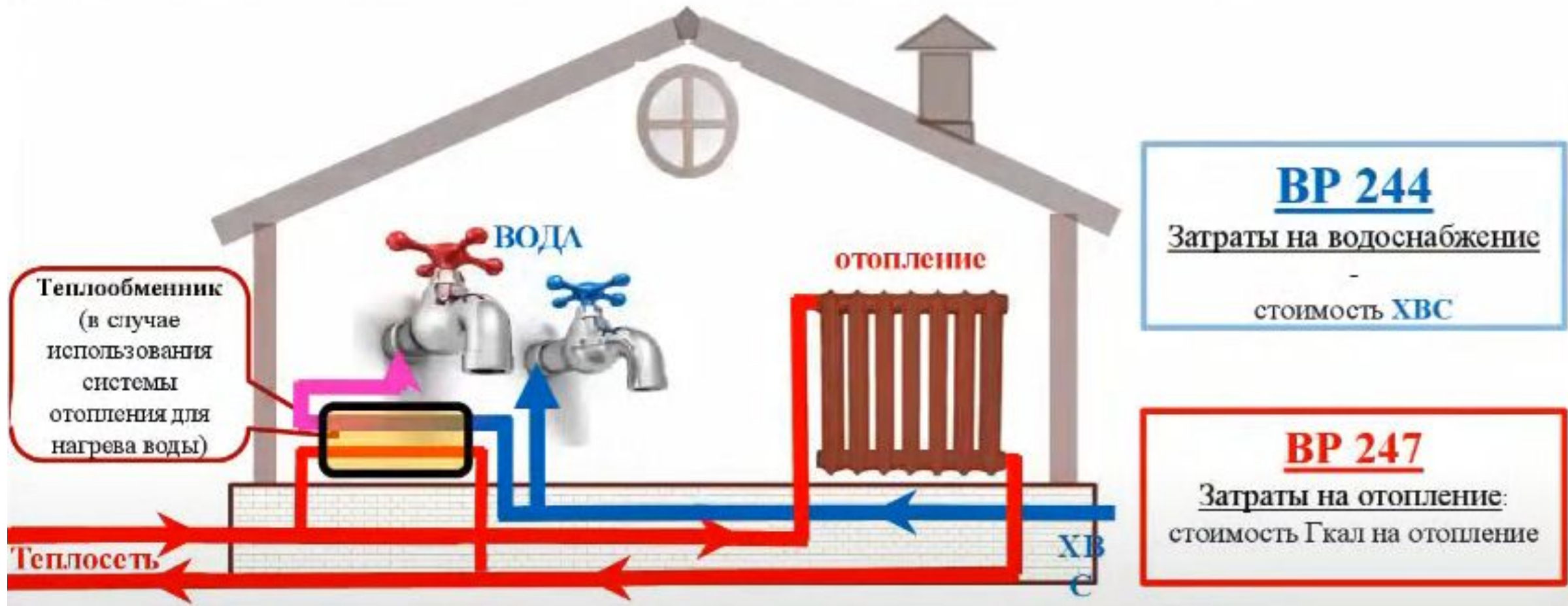
Рисунок 2. Закрытая система теплоснабжения (а)
