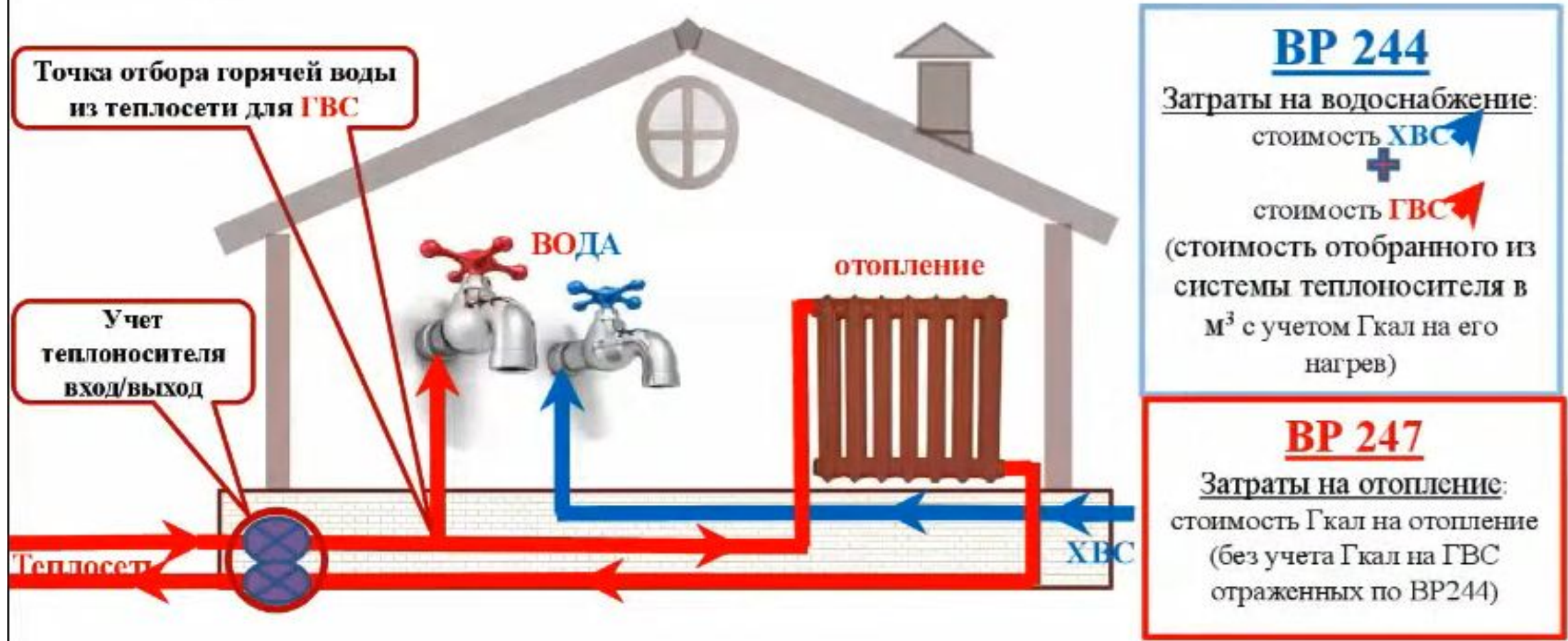
Рисунок 1. Открытая система теплоснабжения
