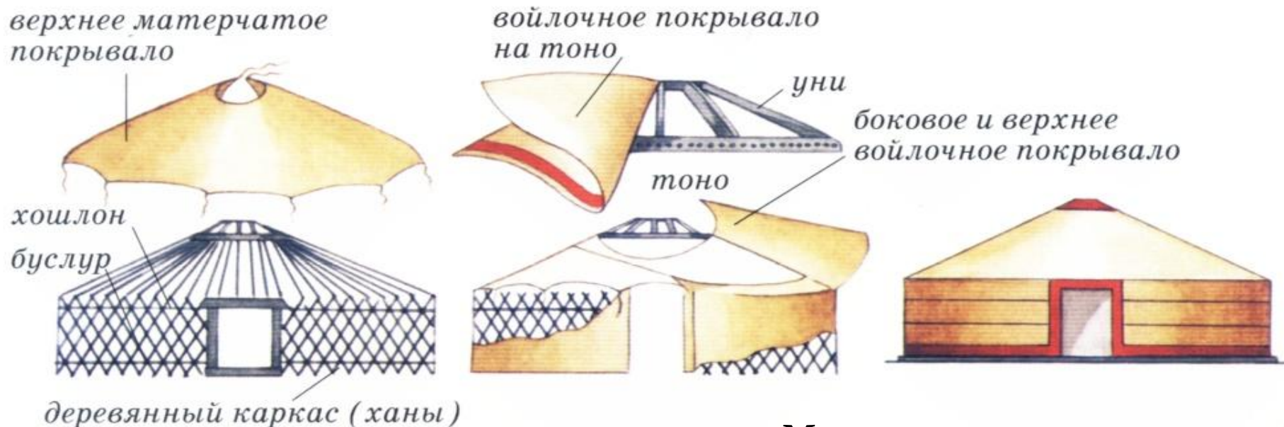
Монгольская юрта
