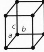
Ромбоэдрическая (тригональная)
