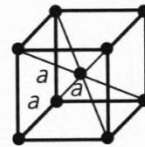
Объемно-центрированная кубическая
