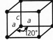
Гексагональная
