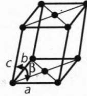
Базоцентрированная моноклинная
