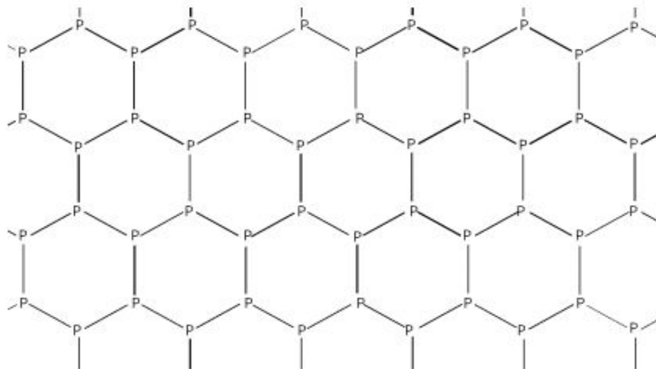
Чёрный фосфор:
