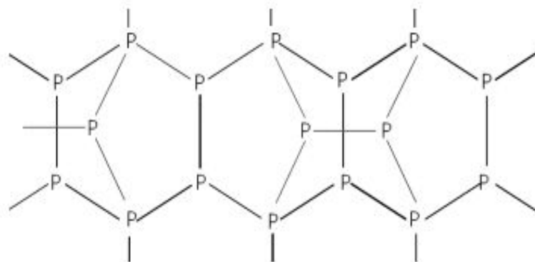
Красный фосфор:
