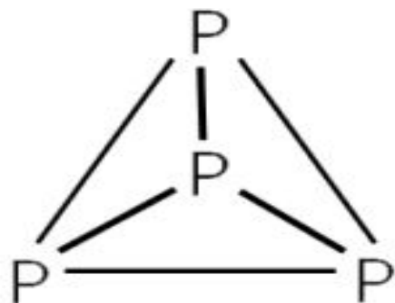
Белый фосфор:
