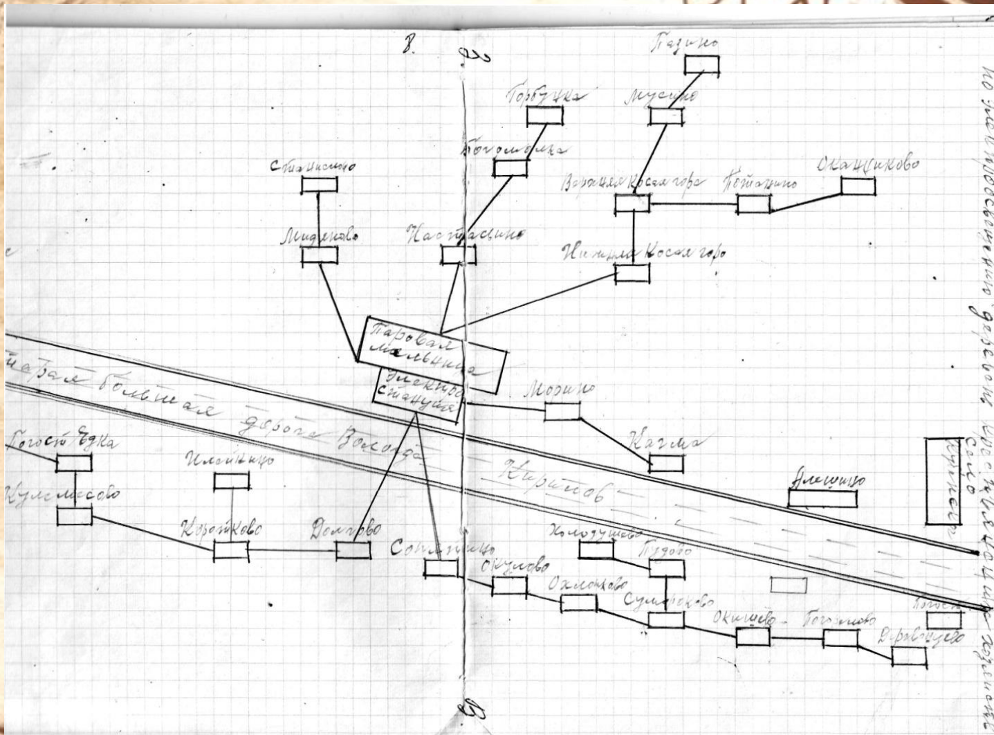
Схема расположения линий электропередач
