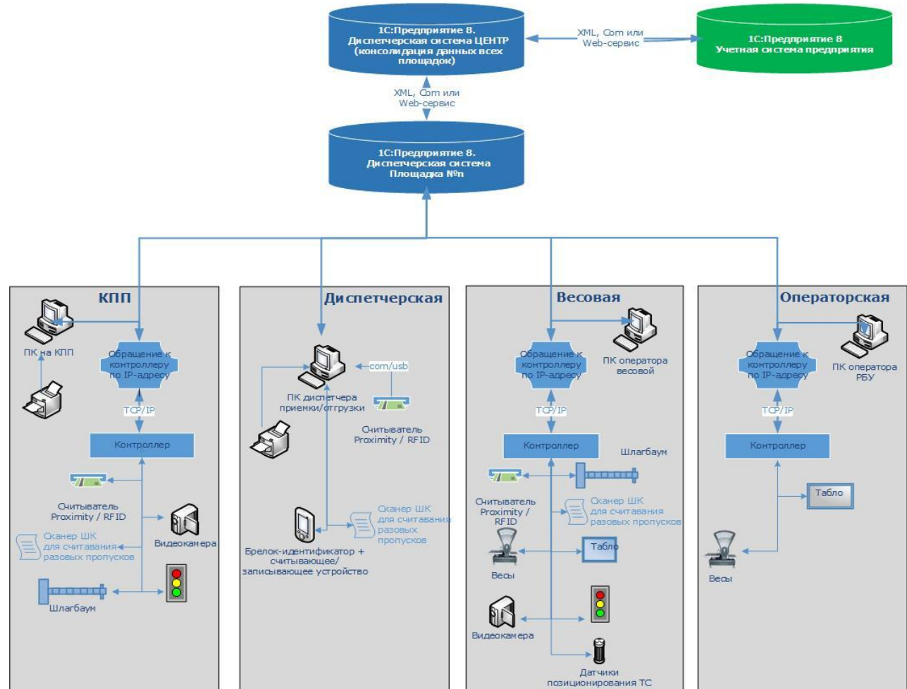
Схема оборудования и АС
