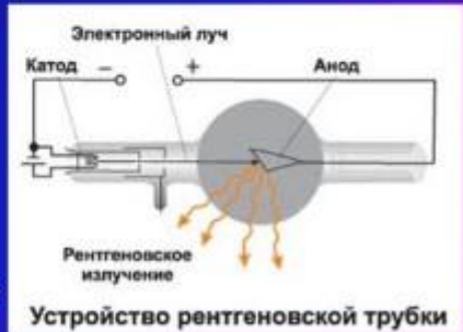
Устройство рентгеновской трубки
