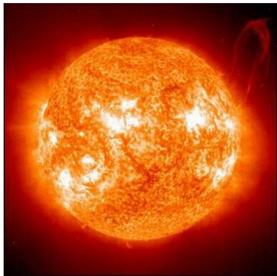
Солнце
