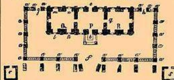
6. Планъ Ледяного дома; а, а—ледяная рѣшетка; б—крыльцо; Р—спяне; Q—лѣвая комната; f—главныйъ ворота; g, h—задняя ворота; m, n, k, l—окна; c—задняя дверь; r, s—пирамиды.
