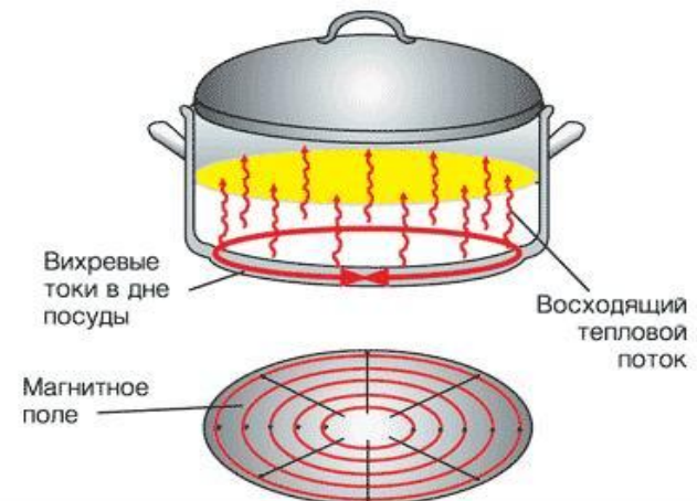
Рис. 3. Индукционная конфорка
