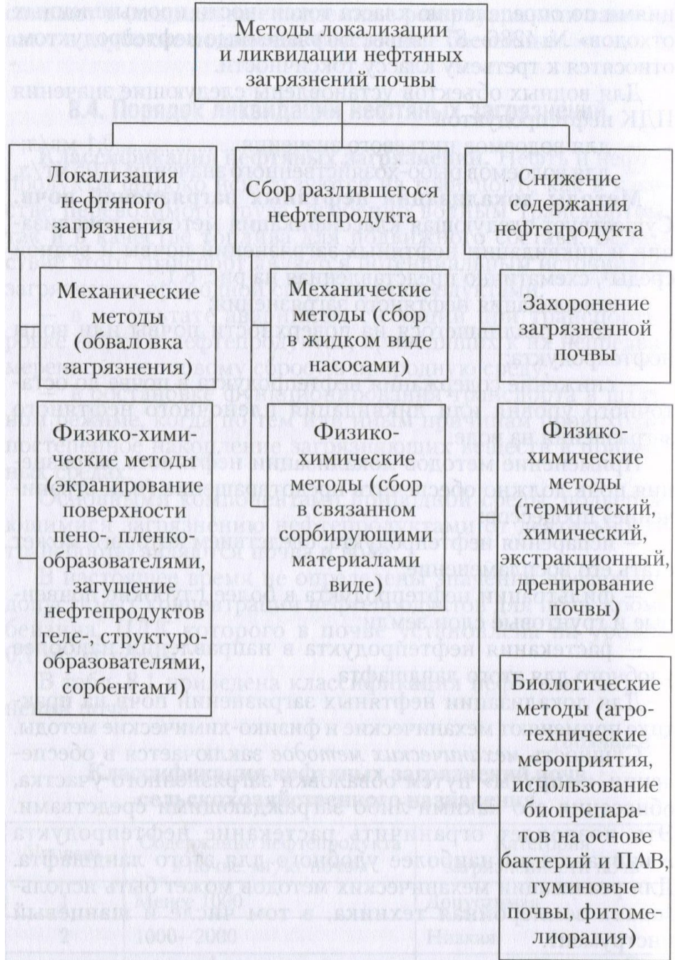
Рис. 8.1. Классификация методов локализации и ликвидации нефтяных загрязнений почвы
