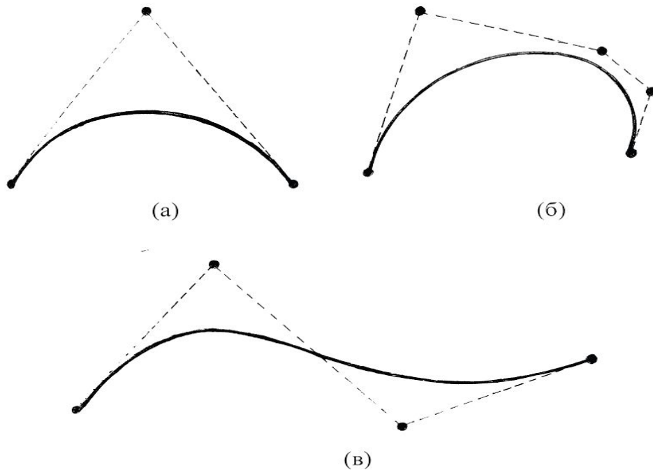
Рис.2.3 Кривые Безье
