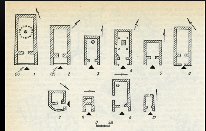
Варианты планов мегаронов
