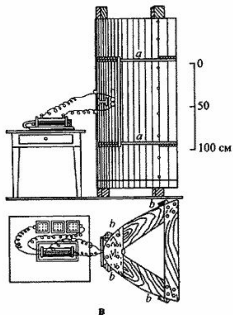
Рис. 5. а – Спирали Рисса с подключенной к ним лейденской банкой, б – вибратор с первичным искровым промежутком (А) и резонатор с вторичным искровым промежутком (В), в – параболическое зеркало с вибратором, связанным проводами с индуктором и батареей (на столике)
