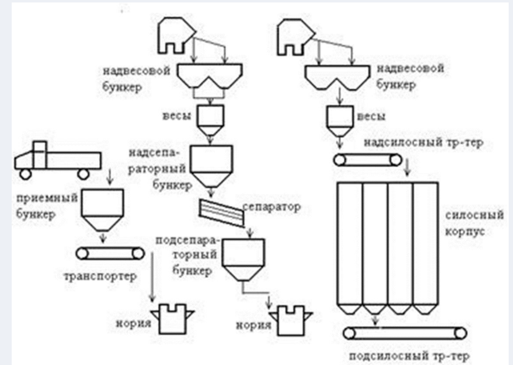
Общая схема приема, хранения и выдачи зерна
