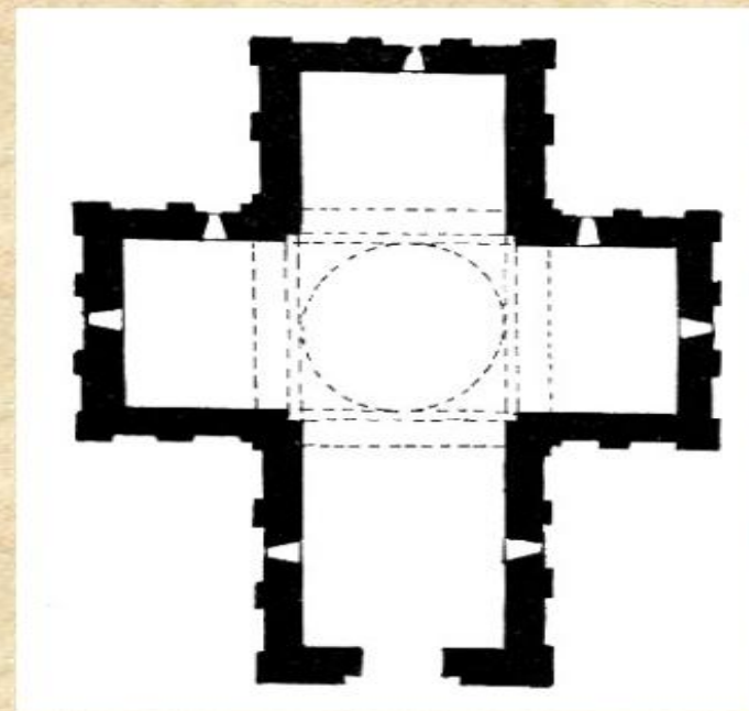
Крестово-купольный храм
